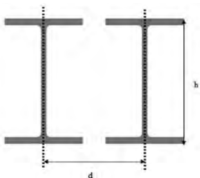
Figura C3.3.28 – Travi parallele
