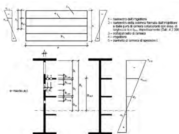
Figura C4.2.16 - Lastra irrigidita pressoinflessa
