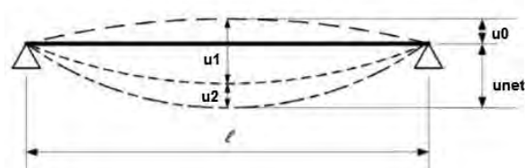
Figura C4.4.1 – Deformazione per un elemento inflesso
