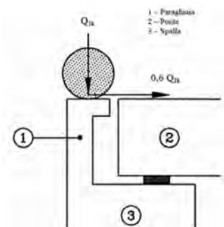
Figura C5.1.1 - Carichi da traffico su muri paraghiaia
