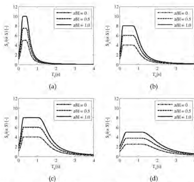
Figura C7.2.4 - Accelerazione massima, normalizzata rispetto ad aS , per i seguenti valori di T_1 : (a) T_1 = 0,3 s, (b) T_1 = 0,6 s, (c) T_1 = 0,9 s, (d) T_1 = 1,2 s.
