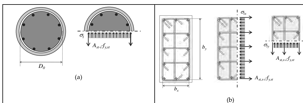
Figura C4.1.7- Pressione laterale di confinamento: (a) sezioni circolari, (b) sezioni rettangolari
